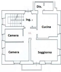
PIANTA PIANO SECONDO
