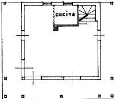
PIANO PRIMO H = 2.60
