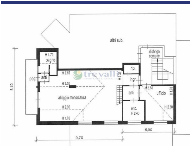
SECONDO PIANO SOTTOSTRADA H ml. 2.50
