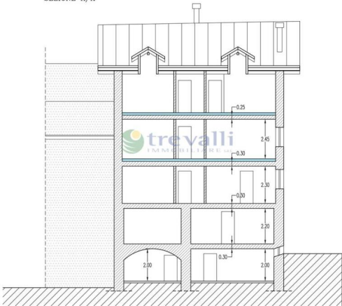
SEZIONE A/A
