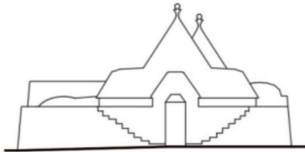
PROSPETTO SUD-EST Scala 1:100
