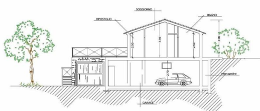
SEZIONE A - A
