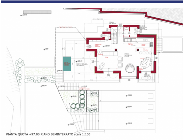
PIANTA QUOTA +97.00 PIANO SEMINTERRATO scala 1:100
