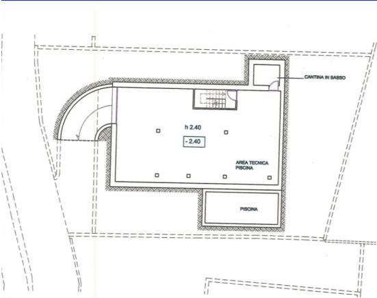
PIANTA PIANO INTERRATO - scala 1:200
